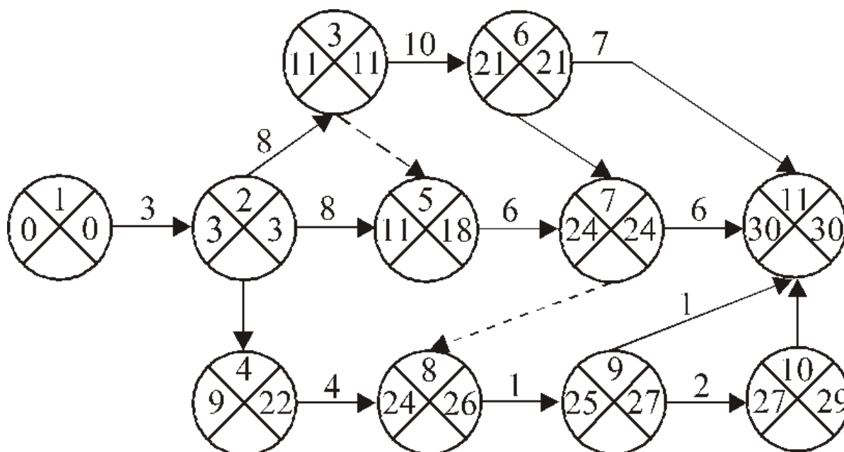
Сетевой график монтажа подстанции 10/04 кВ
